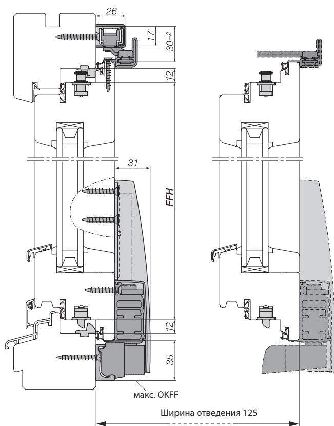
Разрез по вертикали, ATRIUM HKS® 160 S дерево
