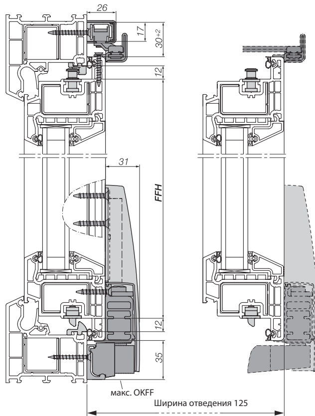
Разрез по вертикали, ATRIUM HKS® 160 S пластик
