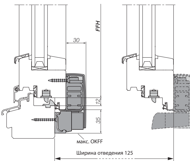
Разрез по вертикали, ATRIUM HKS® 100 S пластик
