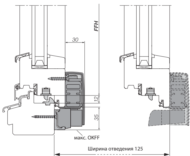
Разрез по вертикали, ATRIUM HKS® 100 S дерево
